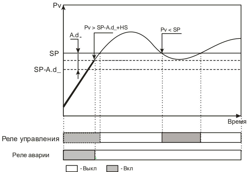
Рис.5 Иллюстрация использования режима оперативного (ручного) отключения реле
