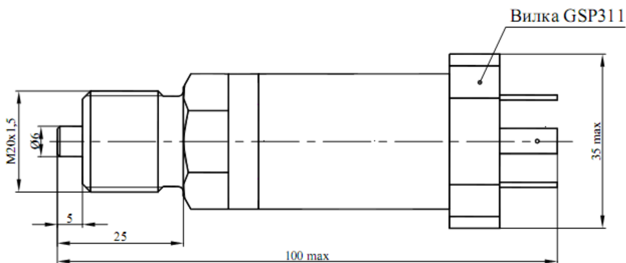
Рисунок В.1 – Габаритный чертеж преобразователей избыточного давления, давления-разрежения со штуцером M20x1,5 и соединительным разъемом DIN 43650 А
