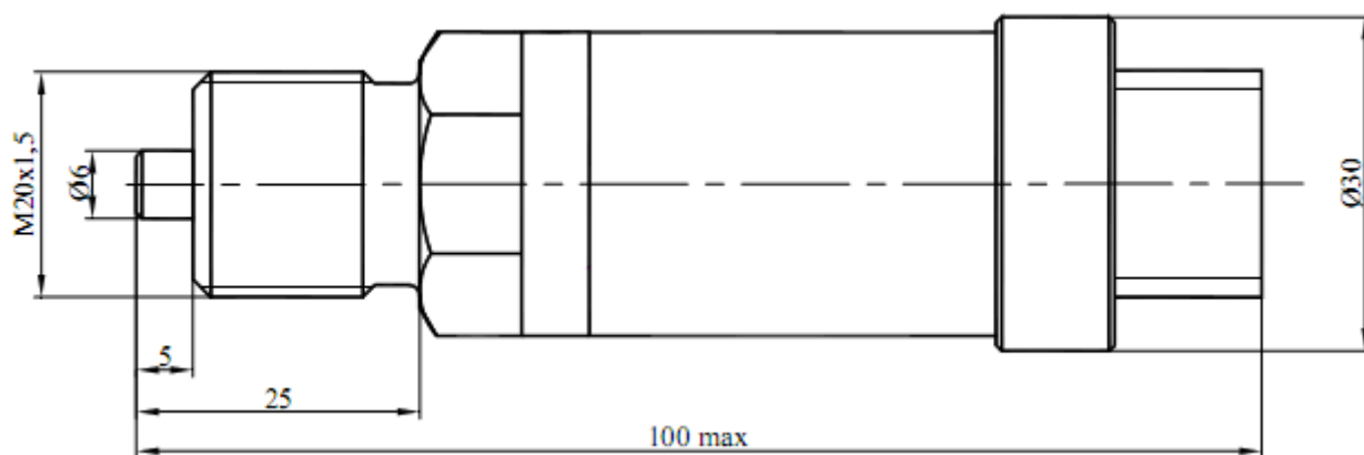
Рисунок В.2 – Габаритный чертеж преобразователей избыточного давления, давления-разрежения со штуцером M20x1,5 и соединительным разъемом 2РМГД18Б4Ш5В1 и 2РМДТ18Б7Ш1В1В
