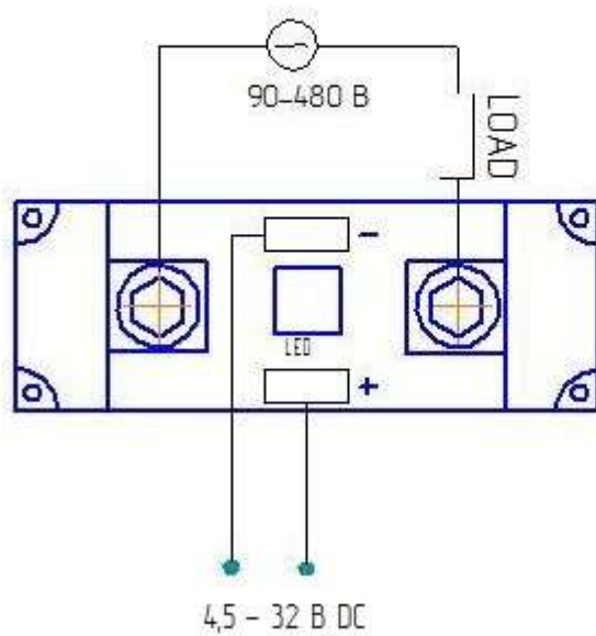
Рисунок 2 – Схема подключения
