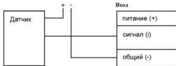
Двухпроводная схема с внешним питанием
