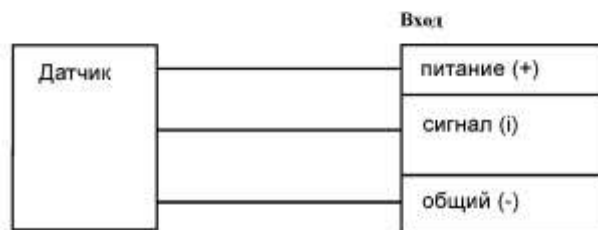
Трёхпроводная схема
