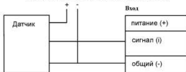
Трёхпроводная схема с внешним питанием
